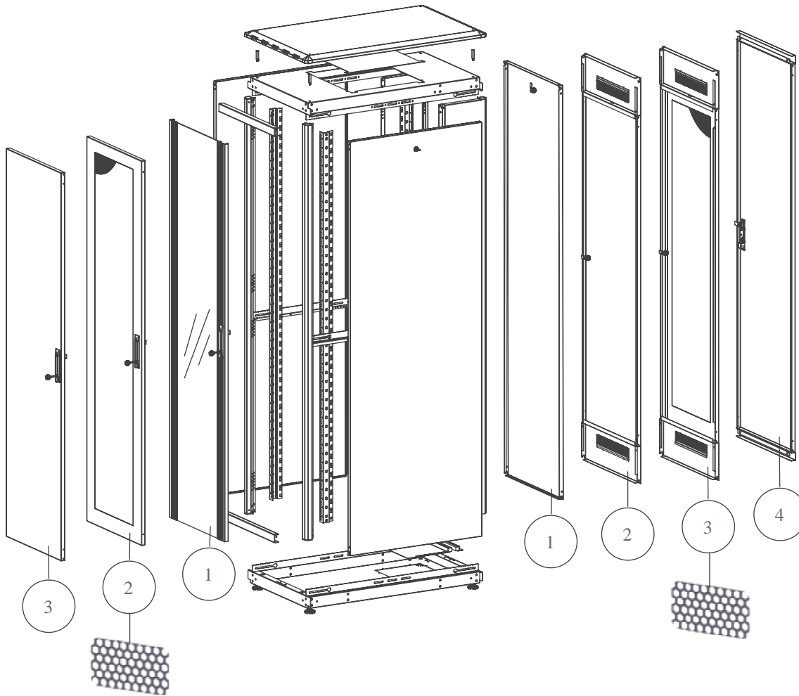
Напольный шкаф DYNAmic Ш=600мм Г=1000мм Все варианты ПЕРЕДНЕЙ ДВЕРИ любой высоты
