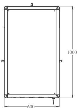
ВИД СВЕРХУ
