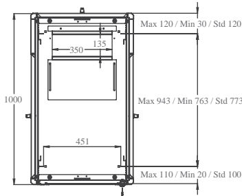
МАКС./СТАНД./МИН. РАССТОЯНИЯ МОНТАЖА ОБОРУДОВАНИЯ
