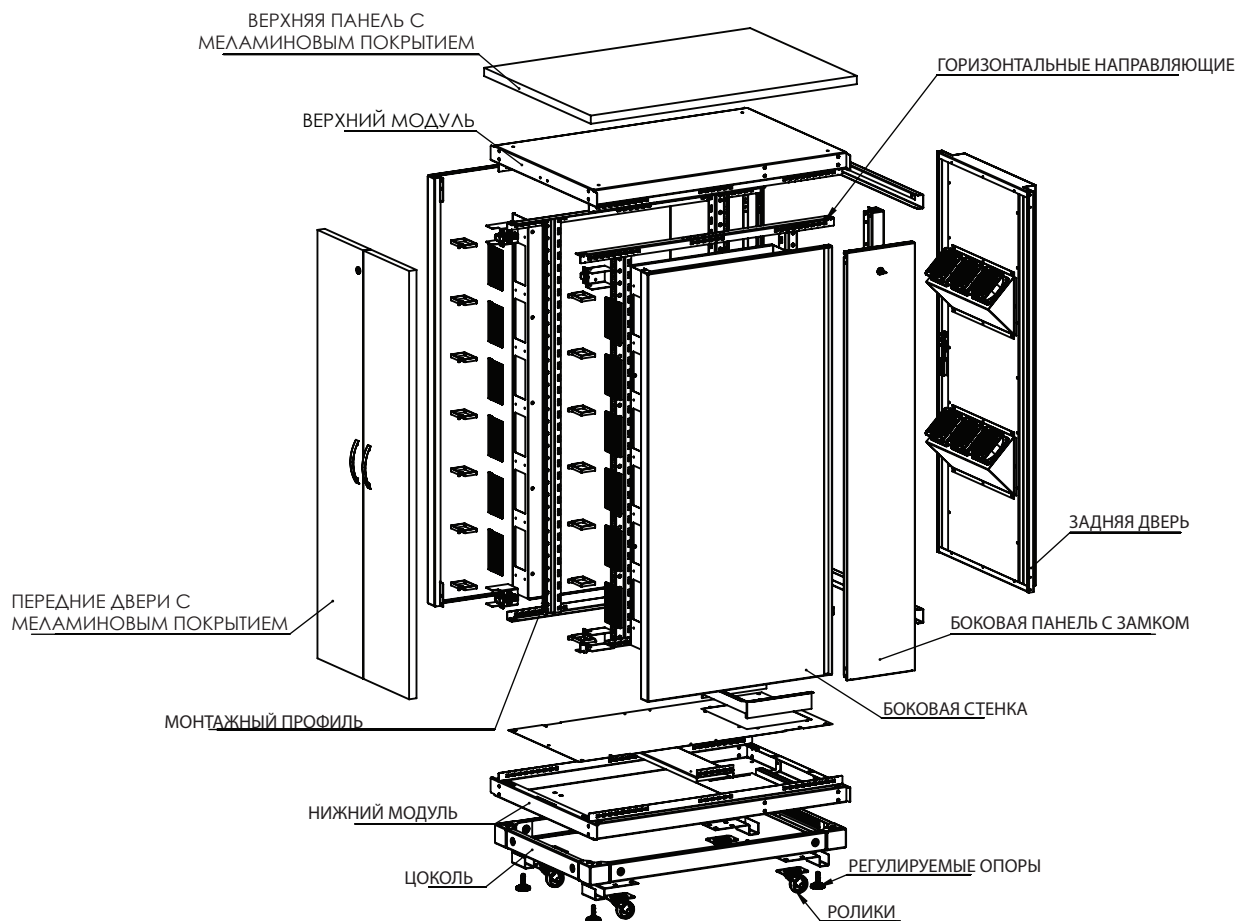
ДЕТАЛЬНЫЙ ВИД
