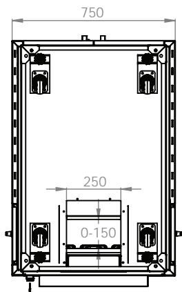
ВИД СНИЗУ
