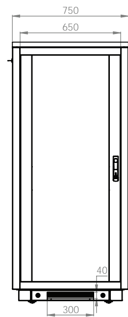
ВИД СЗАДИ
